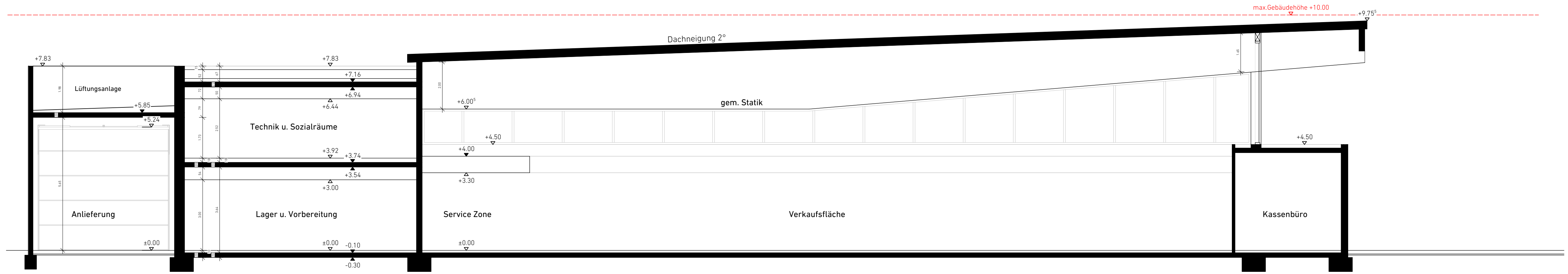
Schnitt A-A Längsschnitt
